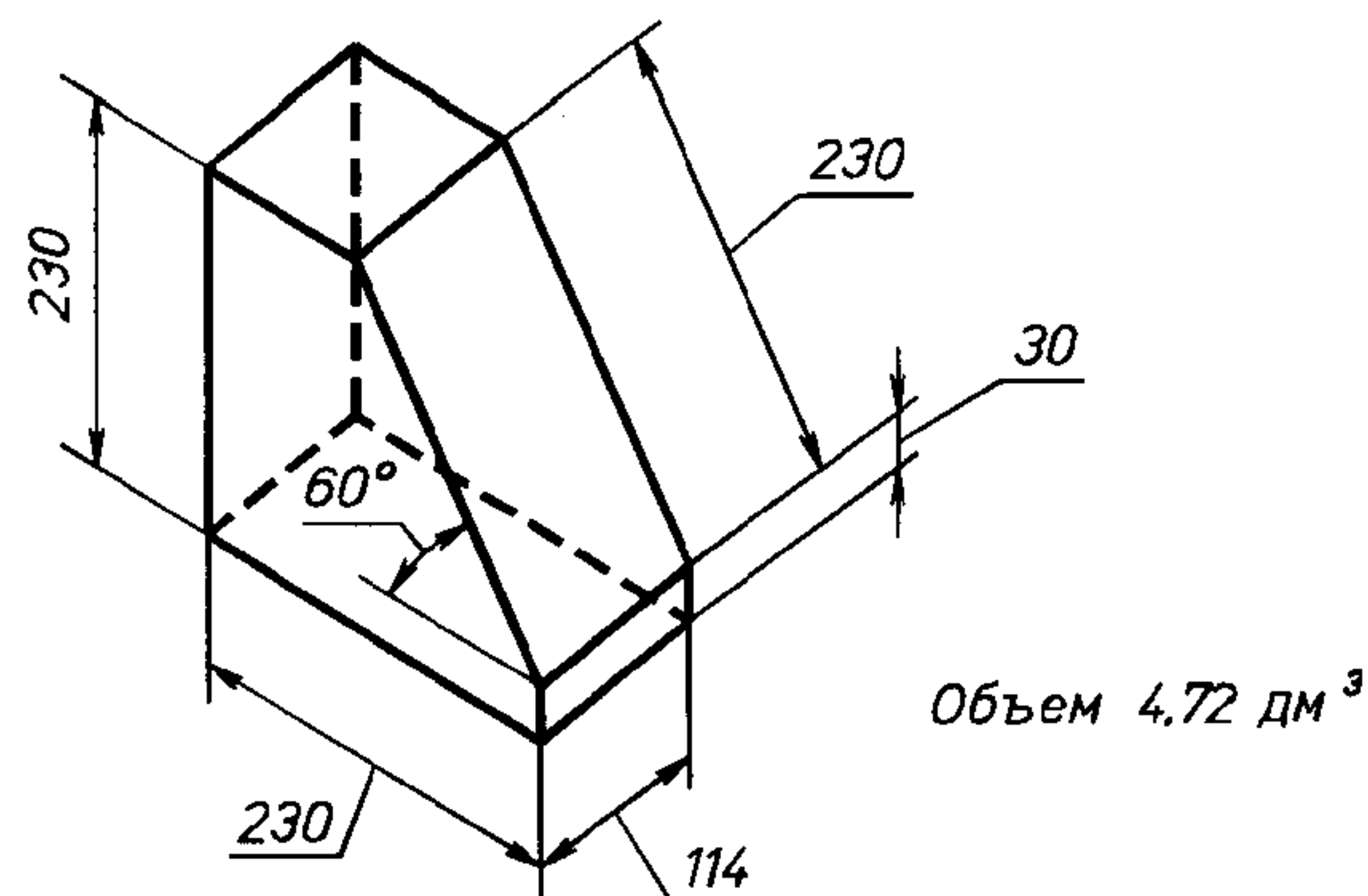
Пятовой кирпич для применения с кирпичом горизонтального ряда кладки высотой 76 мм
